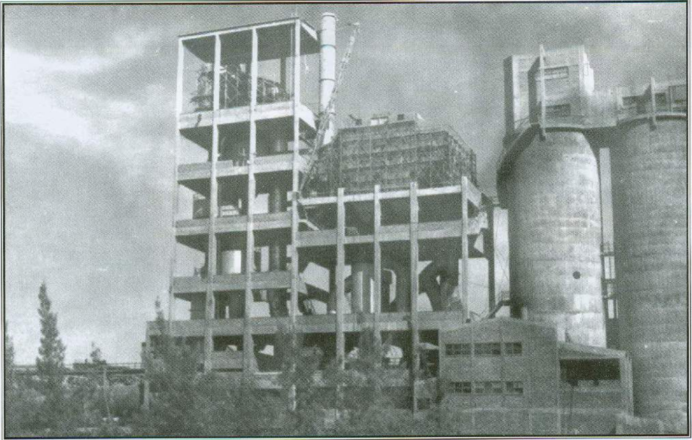
1957 yılında yapılan Çimento Fabrikasının 1968 yılında ilave olarak yapılan ek binasından bir görünüm (Özcan Güneş Arşivi)
