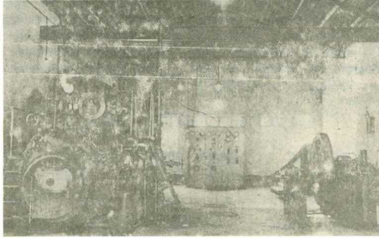
Çorum Belediye elektrik santrali
